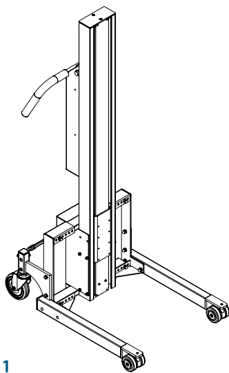
Flexleg type 1 WP 130S/WP 130/WP 130EM/ WP 130EMX/WP 130EMXX
