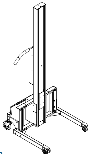
Flexleg type 2 WP 130S/WP 130/WP 130EM/ WP 130EMX/WP 130EMXX
